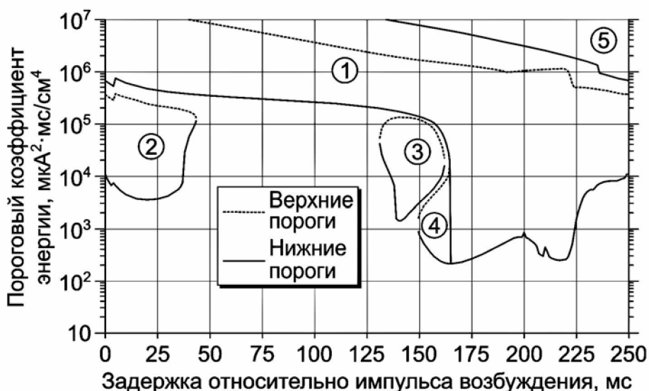
Рис. 3. Зависимость пороговых коэффициентов энергии импульса деполяризации, вызывающих удлинение рефрактерного периода модели кардиомиоцита, от задержки относительно импульса возбуждения при длительности импульса деполяризации 5 мс (1...5 – области эффективности импульса деполяризации)
